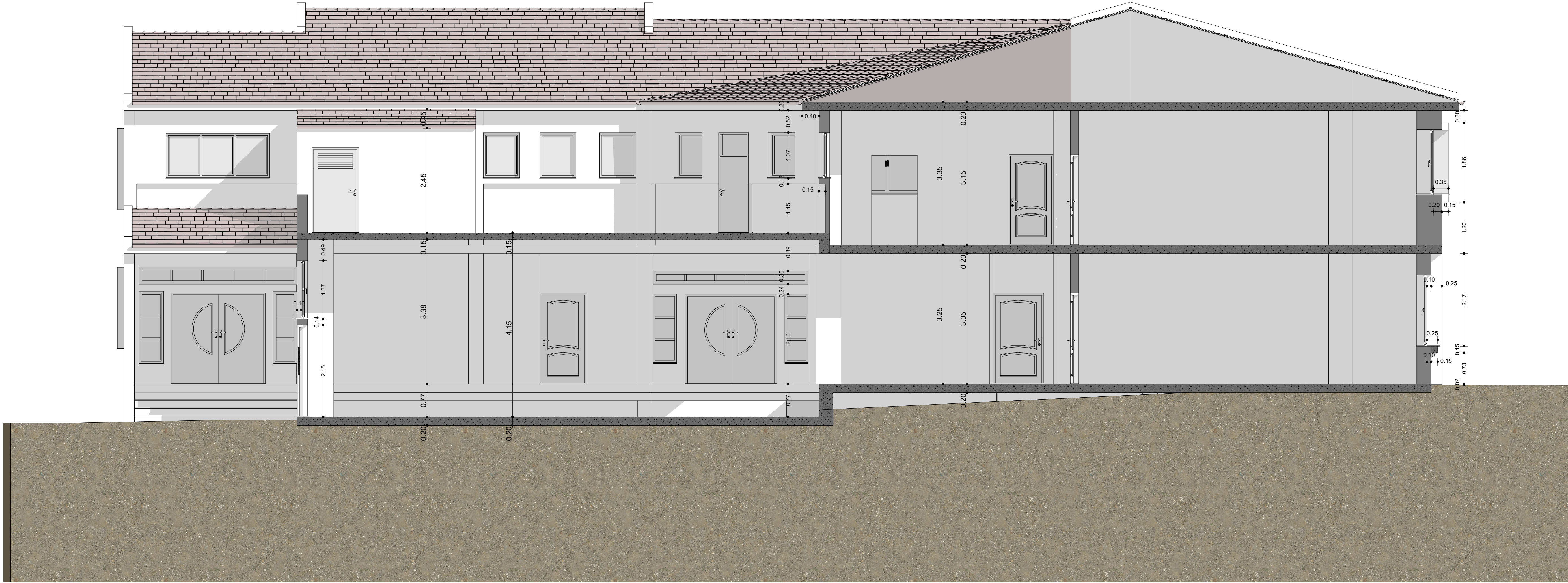
1:50 Τομή Κτηρίου T-03
